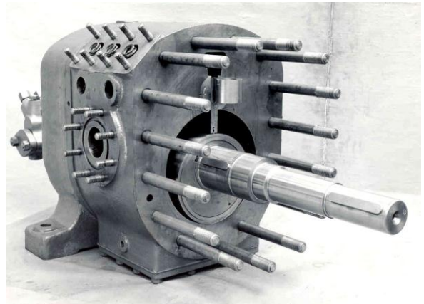
Bild 3: Rotasco-Kompressor der Rathaus-Wärmepumpe [Hochbauamt, Zürich]
