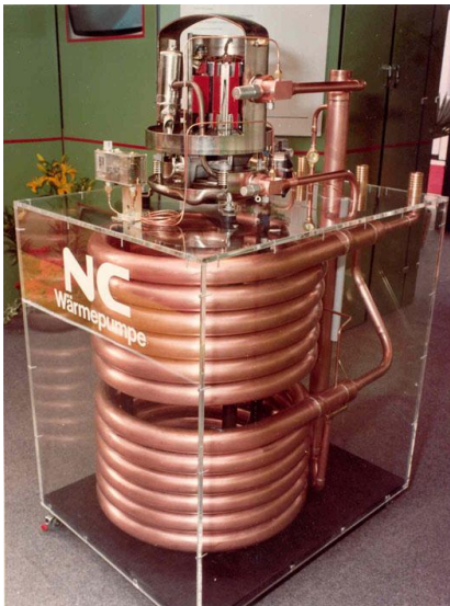
Bild 8: "Grimm Maschine" um 1980 [H. Grimm, Bremgarten]
