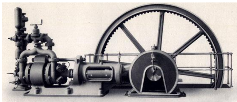
Bild 1: Kolbenkompressor um 1905 [Archiv Sulzer, Winterthur].
