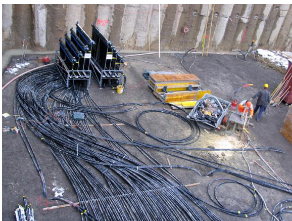
Bild 12: Erdwärmespeicher im Bau, Hotel "The Dolder Grand", Zürich [GEOWATT AG, Zürich]
