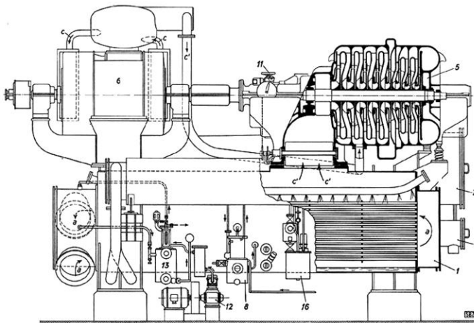
Bild 4: Walche-Anlage, Brown Boveri « Thermoblock » mit Radialkompressoren [Broschüre, Amt für Bundesbauten, Bern, 1988]
