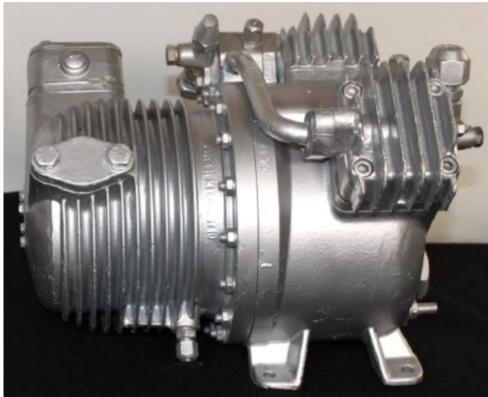
MAB Stirnkurbelverdichter
