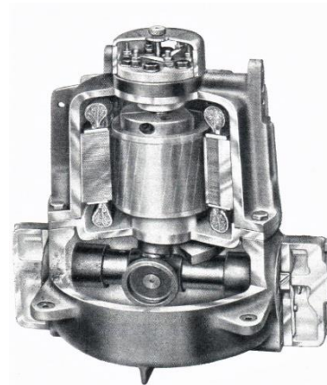
Göldner-Kurbelschleifenverdichter
