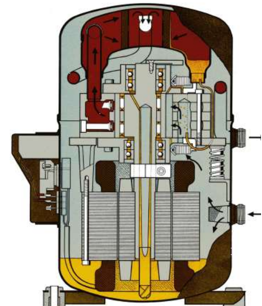
Bitzer HD-20
