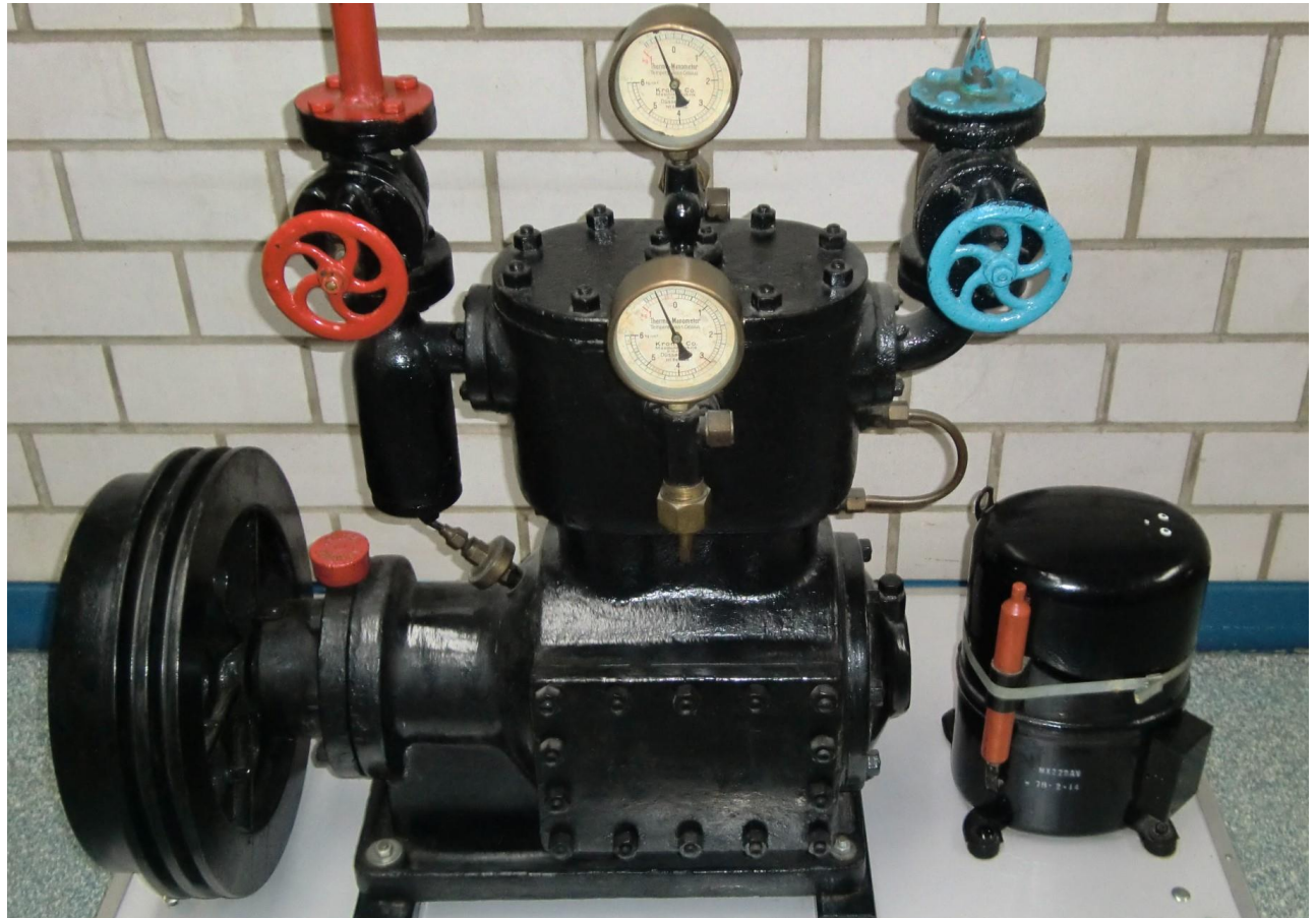
1921 SO 2 Kompressor Metzgerei Kühlraum Kälteleistung :3500 kcal/h bei -10°C VT Antriebsmotor: 3 PS (2,2 kW)
