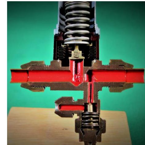
Schnittmodell Saugdruckregler
