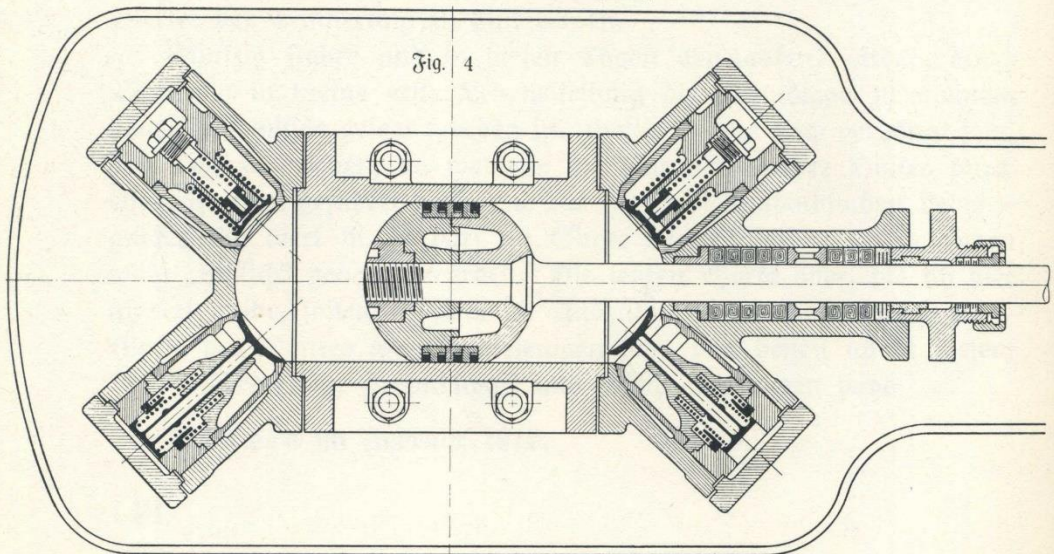
Liegender Ammoniak-Kompressor
