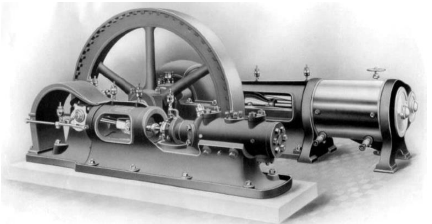
Dampfmaschine gekuppelt mit Kohlendioxid-Kälteverdichter aus Prospekt: Hallesche Maschinenfabrik und Eisgießerei 1935
