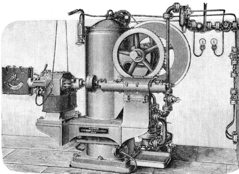
Fig. 2. Elektrisch betriebene Kältemaschine.
